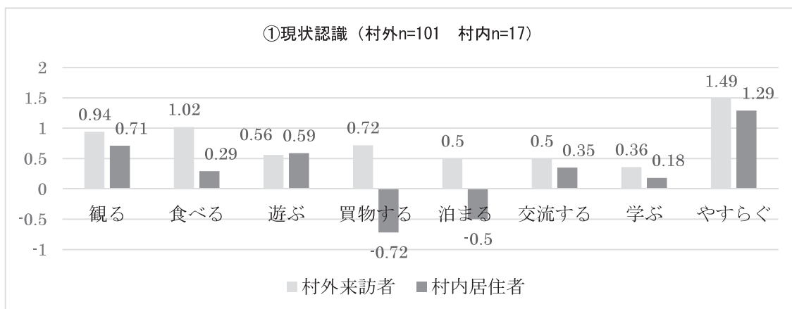
図1 観光の8要素
